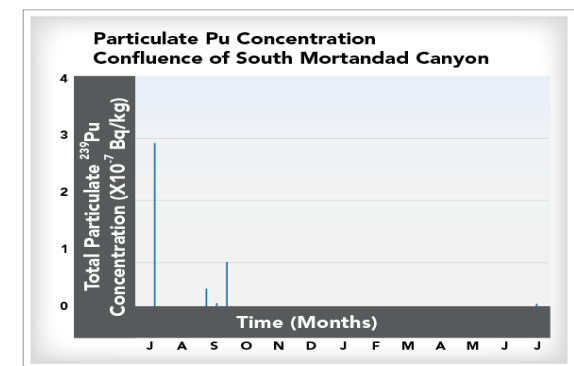
Sediment Sorbed Pu
