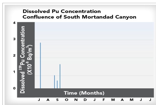
Dissolved Pu
